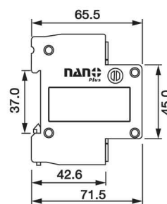
1P+N 10-20 kA
