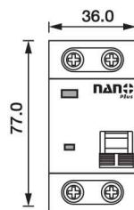
2 Pole 10 kA
