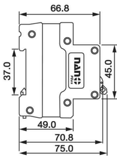
1 Pole 6 kA
