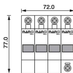
3P+N 10-20 kA
