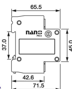
3P+N 10-20 kA
