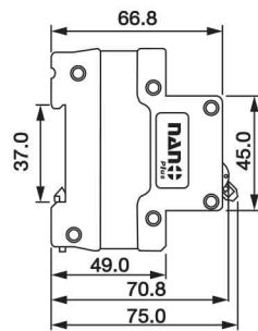
2 Pole 10 kA
