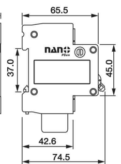
2 Pole 10 kA
