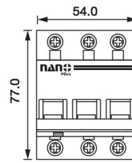
3 Pole 6 kA
