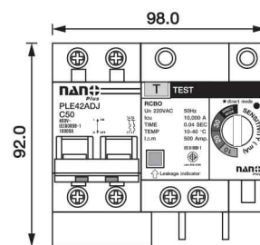
2 Pole 10 kA
