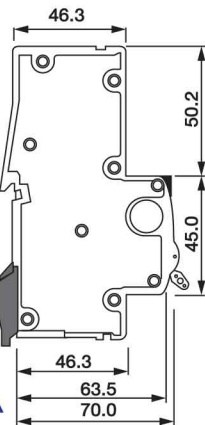
1 Pole 6 kA
