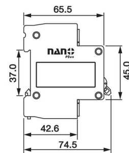
2 Pole 10 kA
